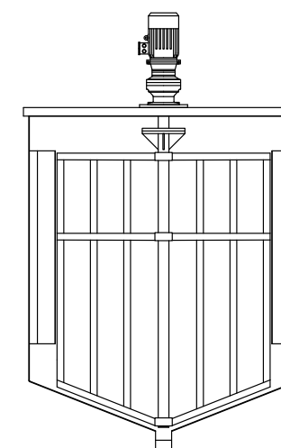
Batteria di vasche costruite in acciaio inox con agitatore a rastrello. Tanks battery built in stainless steel with rake stirrer. Batería de tanques construidas en acero inoxidable con agitador de rastrillo. Batterie de cuves construites en acier inoxydable avec agitateur à râteau.
