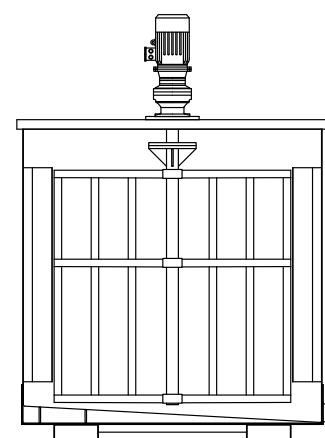
Vasca con fondo inclinato. Tank with inclined bottom. Tanque con fondo inclinado. Cuve avec fond incliné.
