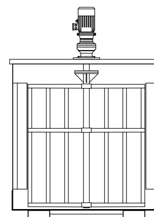
Vasca con fondo pari. Tank with flat bottom. Tanque con fondo plano. Cuve avec fond plat.
