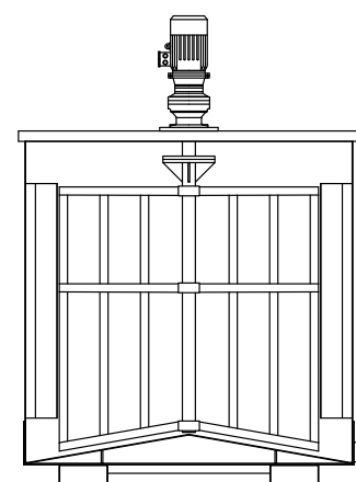
Vasca con fondo conico convesso. Tank with convex conical bottom. Tanque con fondo cónico convexo. Cuve avec fond conique convexe.
