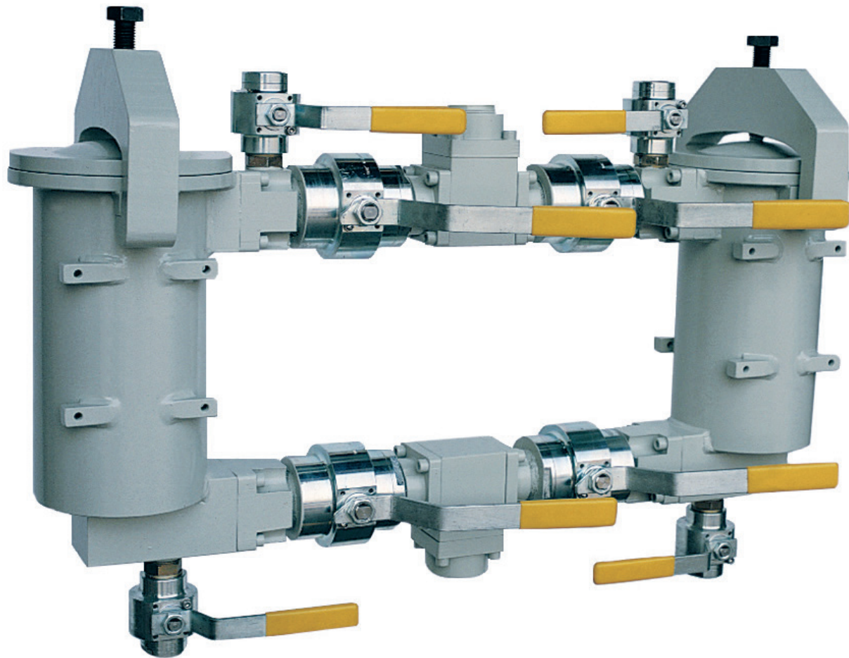
Filtro tipo CFS-M manuale. Manual filter CFS-M type. Filtro tipo CFS-M manual. Filtre type CFS-M manuel.
