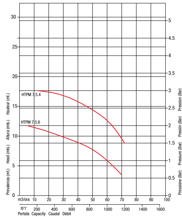
HTPM - Curve con BARBOTTINA 1,7 kg/dm³ HTPM - Curves with SLIP 1.7 kg/dm³ HTPM - Curvas con BARBOTINA 1,7 kg/dm³ HTPM - Courbes avec BARBOTINE 1,7 kg/dm³
