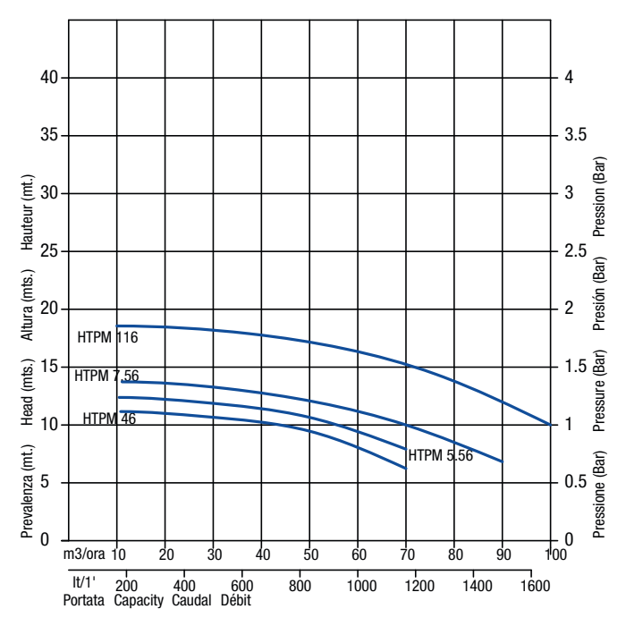
HTPM - Curve con ACQUA 960 rpm HTPM - Curves with WATER 960 rpm HTPM - Curvas con AGUA 960 rpm HTPM - Courbes avec EAU 960 rpm
