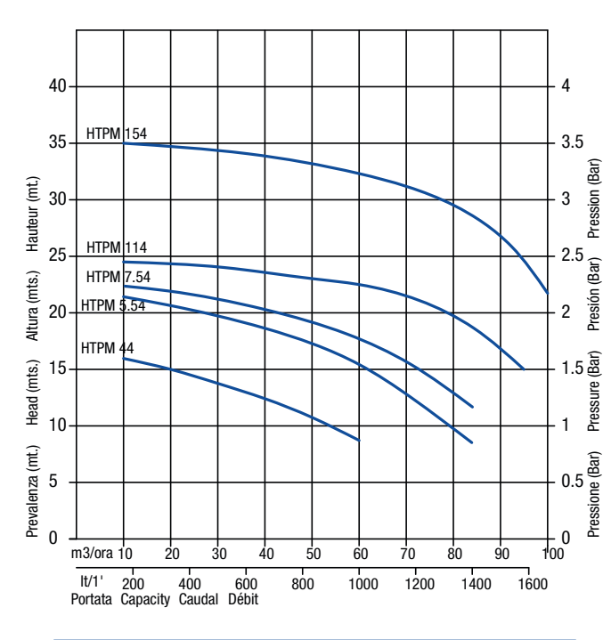
HTPM - Curve con ACQUA 1450 rpm HTPM - Curves with WATER 1450 rpm HTPM - Curvas con AGUA 1450 rpm HTPM - Courbes avec EAU 1450 rpm
