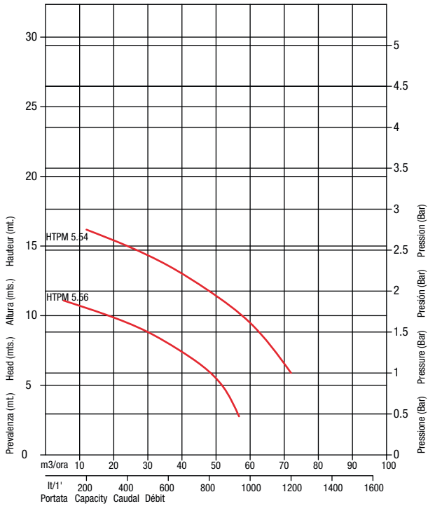
HTPM - Curve con BARBOTTINA 1,7 kg/dm³ HTPM - Curves with SLIP 1.7 kg/dm³ HTPM - Curvas con BARBOTINA 1,7 kg/dm³ HTPM - Courbes avec BARBOTINE 1,7 kg/dm³
