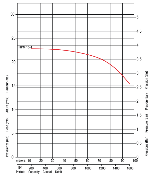
HTPM - Curve con BARBOTTINA 1,7 kg/dm 3 HTPM - Curves with SLIP 1.7 kg/dm 3 HTPM - Curvas con BARBOTINA 1,7 kg/dm 3 HTPM - Courbes avec BARBOTINE 1,7 kg/dm 3
