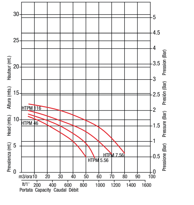
HTPM - Curve con BARBOTTINA 960 rpm 1,7 kg/dm³ HTPM - Curves with SLIP 960 rpm 1.7 kg/dm³ HTPM - Curvas con BARBOTINA 960 rpm 1,7 kg/dm³ HTPM - Courbes avec BARBOTINE 960 rpm 1,7 kg/dm³
