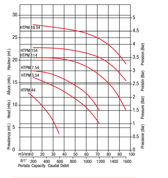
HTPM - Curve con BARBOTTINA 1450 rpm 1,7 kg/dm³ HTPM - Curves with SLIP 1450 rpm 1.7 kg/dm³ HTPM - Curvas con BARBOTINA 1450 rpm 1,7 kg/dm³ HTPM - Courbes avec BARBOTINE 1450 rpm 1,7 kg/dm³
